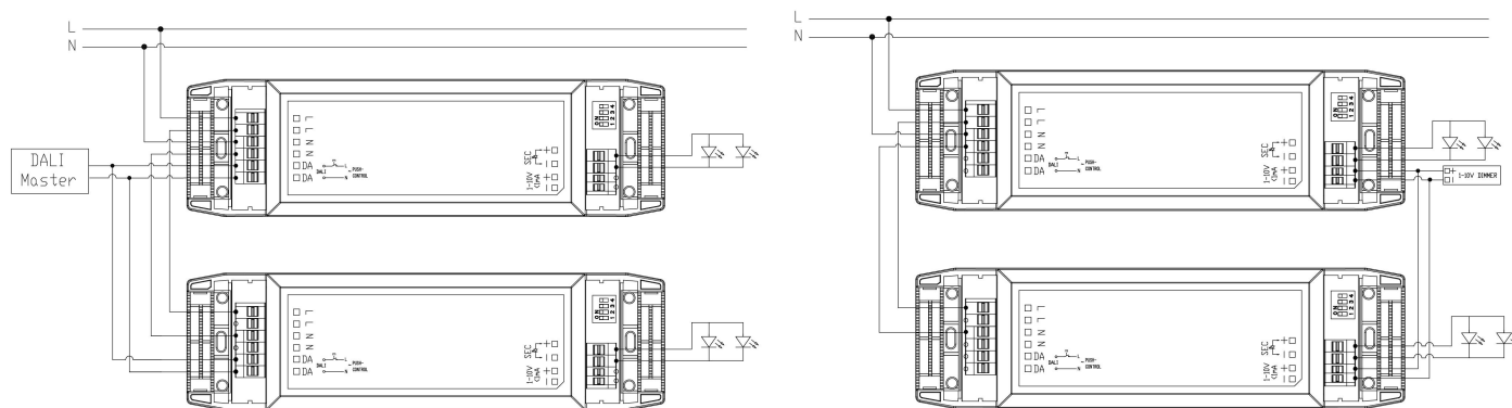
Fig. B DALI Dimming
