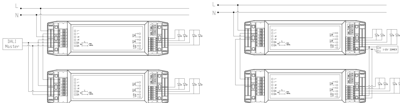
Fig. B DALI Dimming
