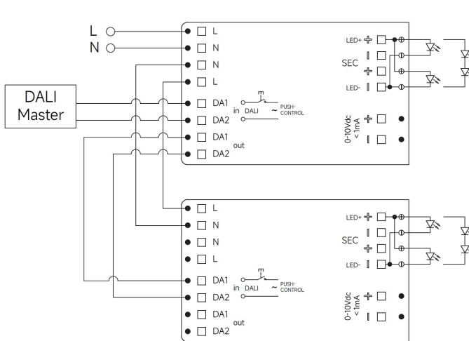
Fig. C: DALI Dimming
