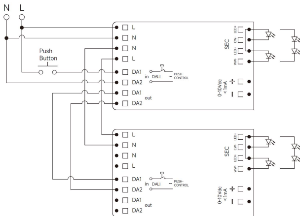
Fig. A: Push Dimming (Parallel)
