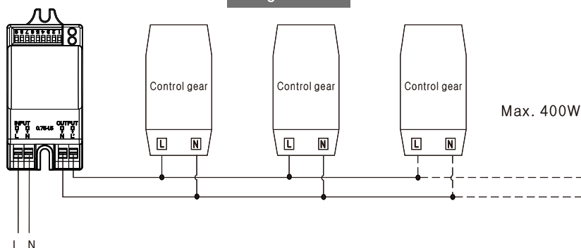
Wiring scheme
