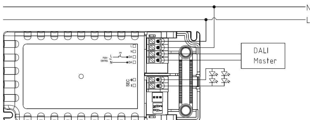
Fig.B DALI Dimming
