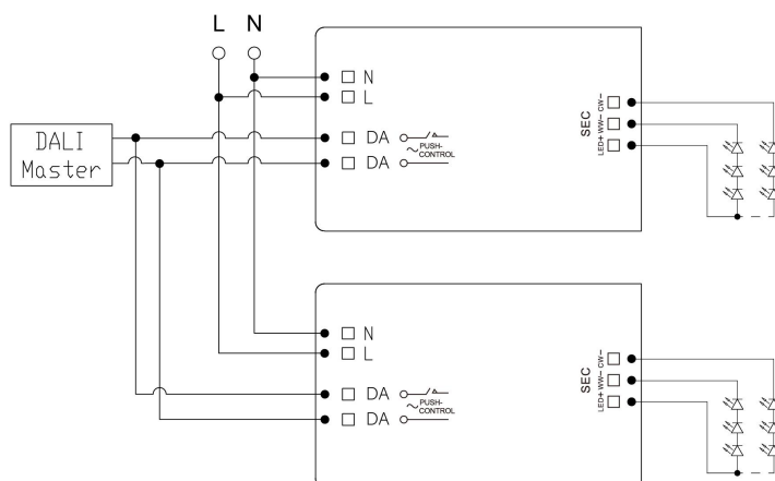
Fig.A DALI Dimming
