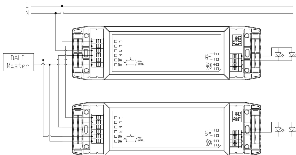
Fig.B DALI Dimming
