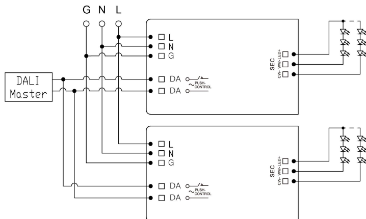
Fig.A DALI Dimming
