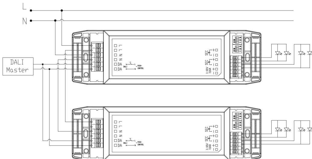
Fig.B DALI Dimming
