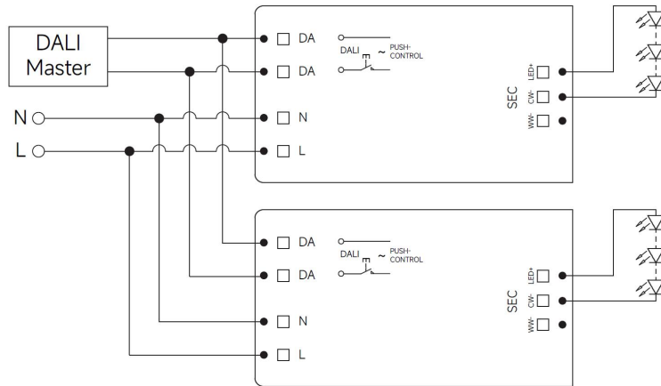
Fig. C: DALI Dimming
