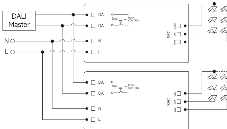
Fig. C: DALI Dimming
