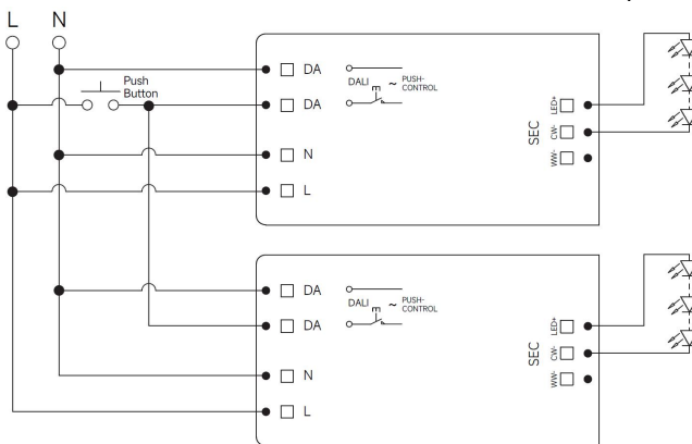
Fig. A: Push Dimming (Parallel)
