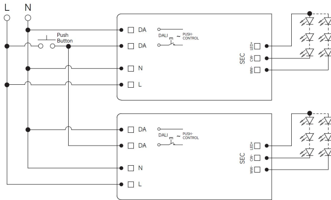
Fig. A: Push Dimming (Parallel)
