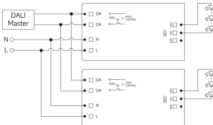
Fig. C: DALI Dimming
