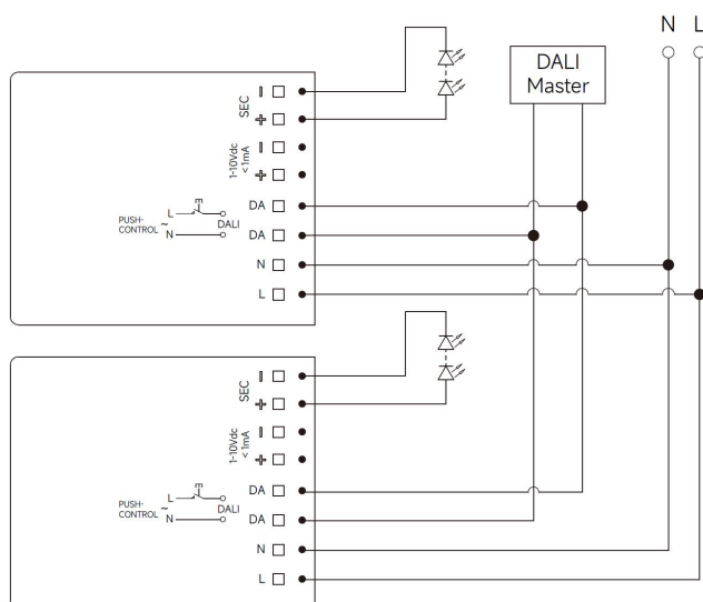
Fig. C: DALI Dimming
