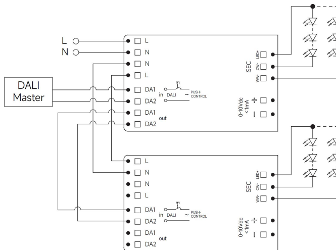
Fig. C: DALI Dimming
