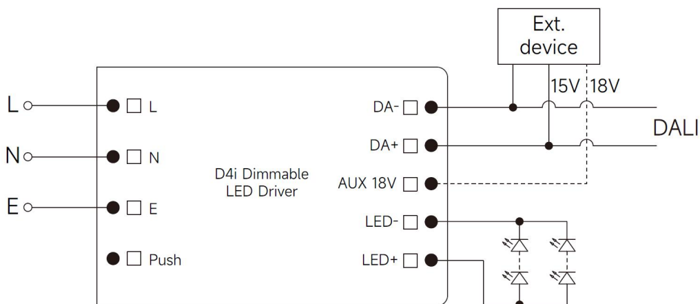
Fig. A: DALI Dimming
