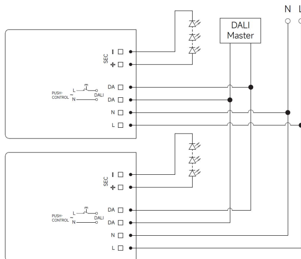
Fig. C: DALI Dimming
