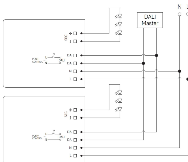
Fig. C: DALI Dimming
