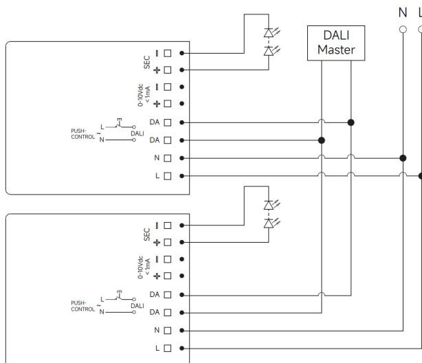
Fig. C: DALI Dimming
