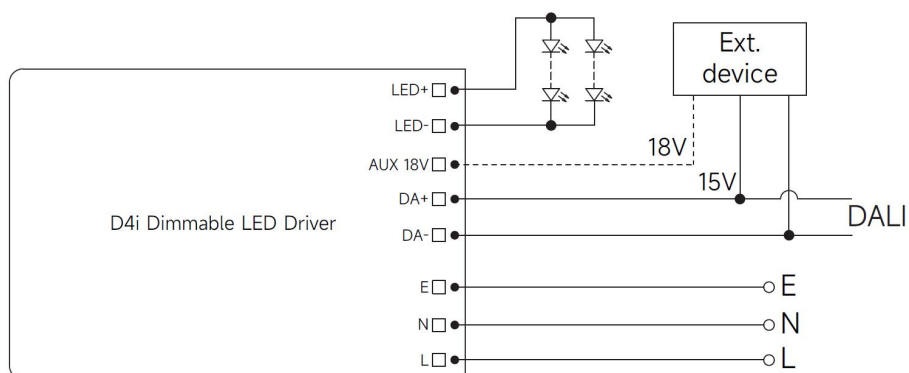
Fig. A: DALI Dimming
