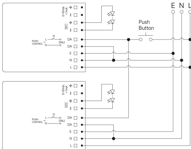
Fig. A: Push Dimming (Parallel)
