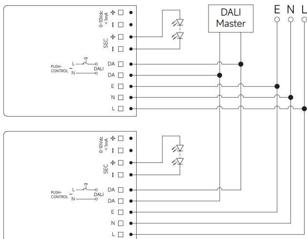
Fig. C: DALI Dimming
